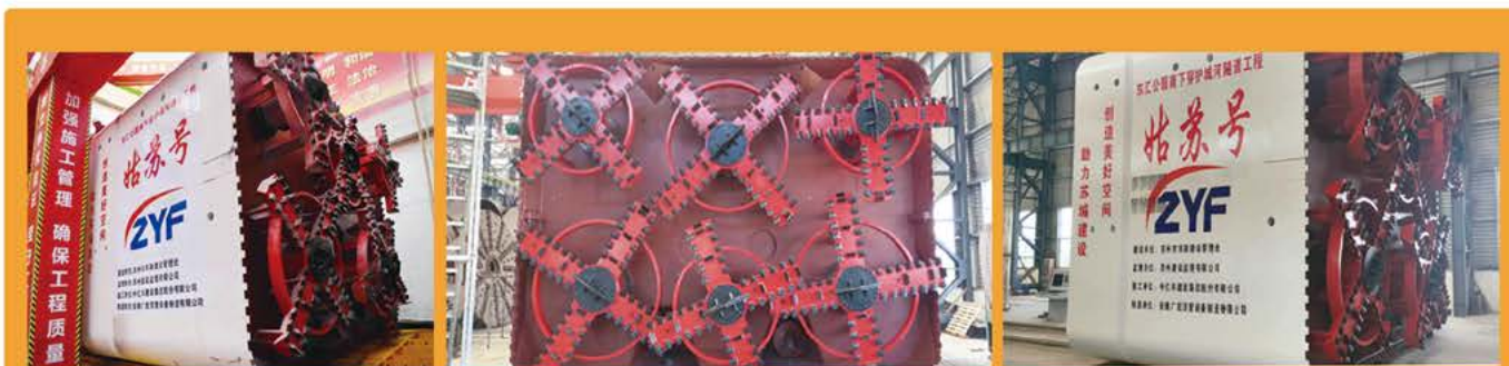
6.9*5.0m多刀盘土压平衡矩形顶管机
